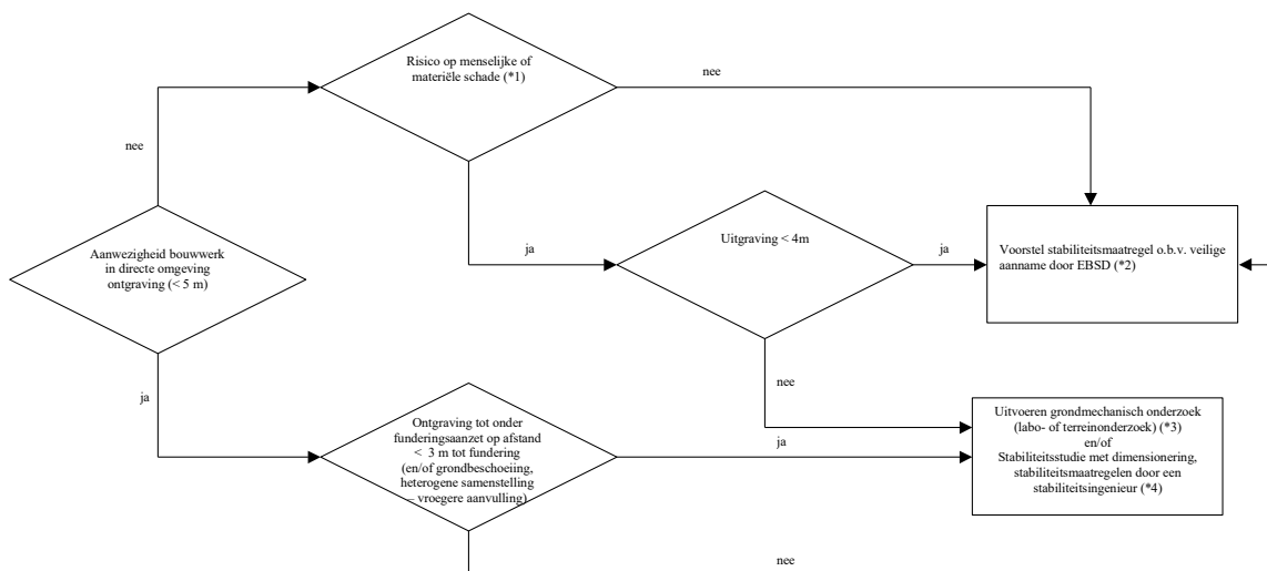
Figuur 1: Beoordelingschema uitgravingsprocedure
